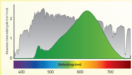
Das naturnahe Lichtspektrum der Pure-Z-NEO-LED Grauer Graph: Spektrum des natürlichen Tageslichts Grüner Graph: Typ. Spektrum der Pure-Z-Retro-LED
