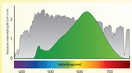
Das naturnahe Lichtspektrum der Pure-Z-NEO-LED Grauer Graph: Spektrum des natürlichen Tageslichts Grüner Graph: Typ. Spektrum der Pure-Z-Retro-LED
